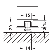
Podlahové vedení s vodicí kolejničkou ve tvaru U a kolečkem podlahového vedení
